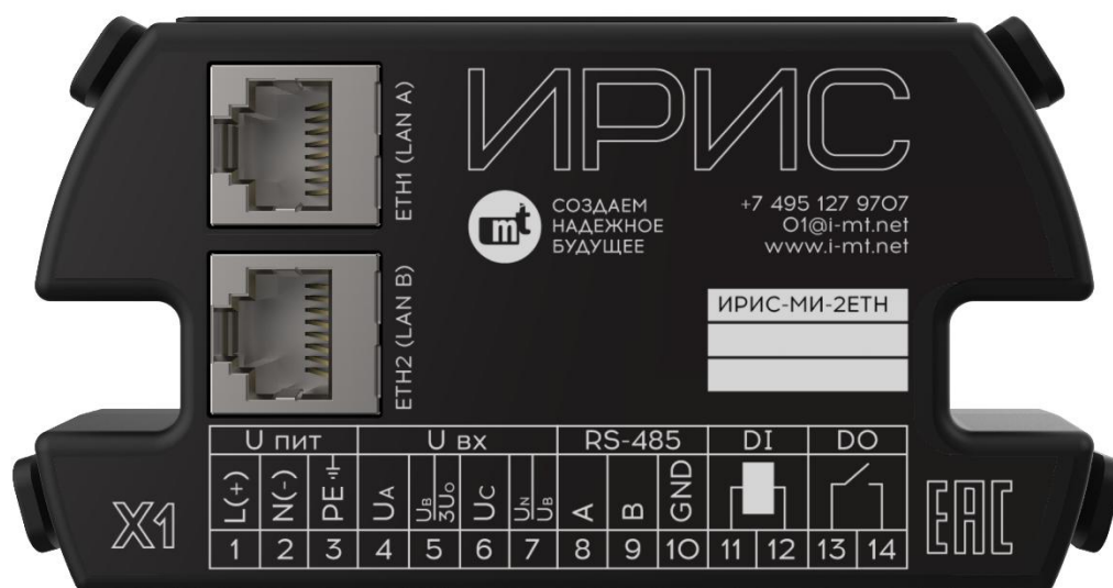
Рисунок 12.11 - Внешний вид рюкзака ИРИС-МИ-2ETH
