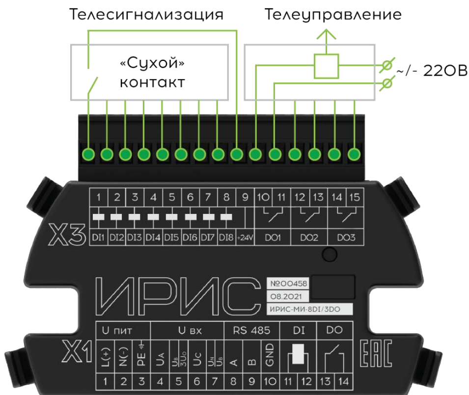
Рисунок 12.7 - Схема подключения рюкзака ИРИС - 8DI/3DO-24V
