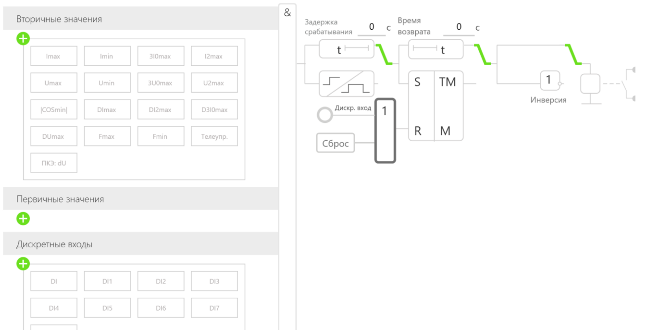
Рисунок 4.2 - Алгоритм работы дискретного выхода
