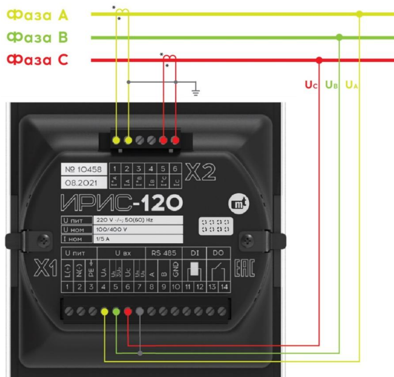
Рисунок 10.3 - Схема подключения устройства с внешними трансформаторами тока и трансформаторами напряжения (2ТТ, 3ТН)
