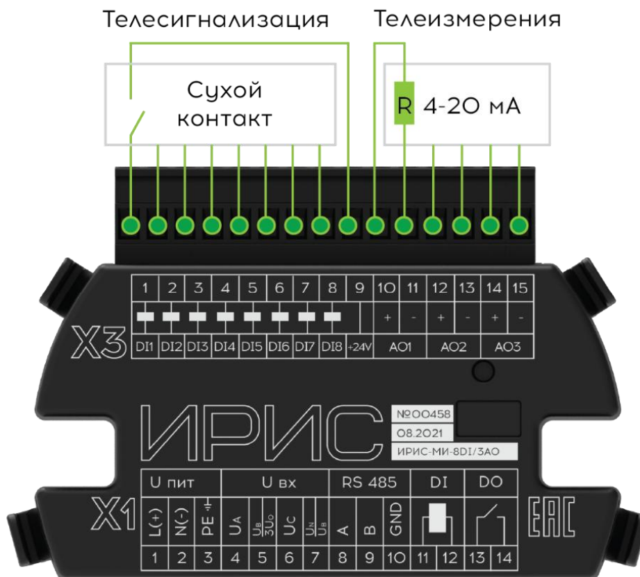
Рисунок 12.9 - Схема подключения рюкзака ИРИС - 8DI/3АО
