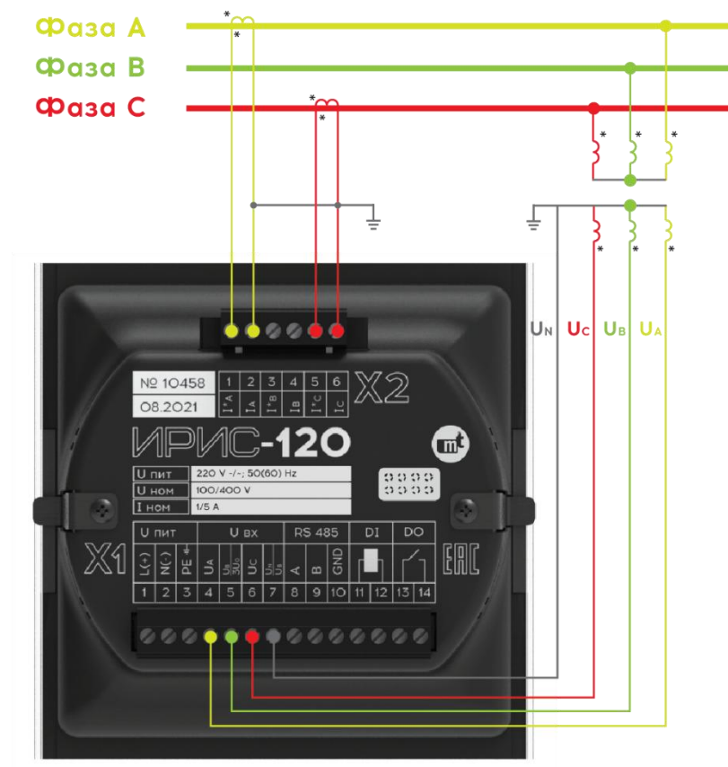
Рисунок 10.3 - Схема подключения устройства с внешними трансформаторами тока и трансформаторами напряжения (2ТТ, 3ТН)
