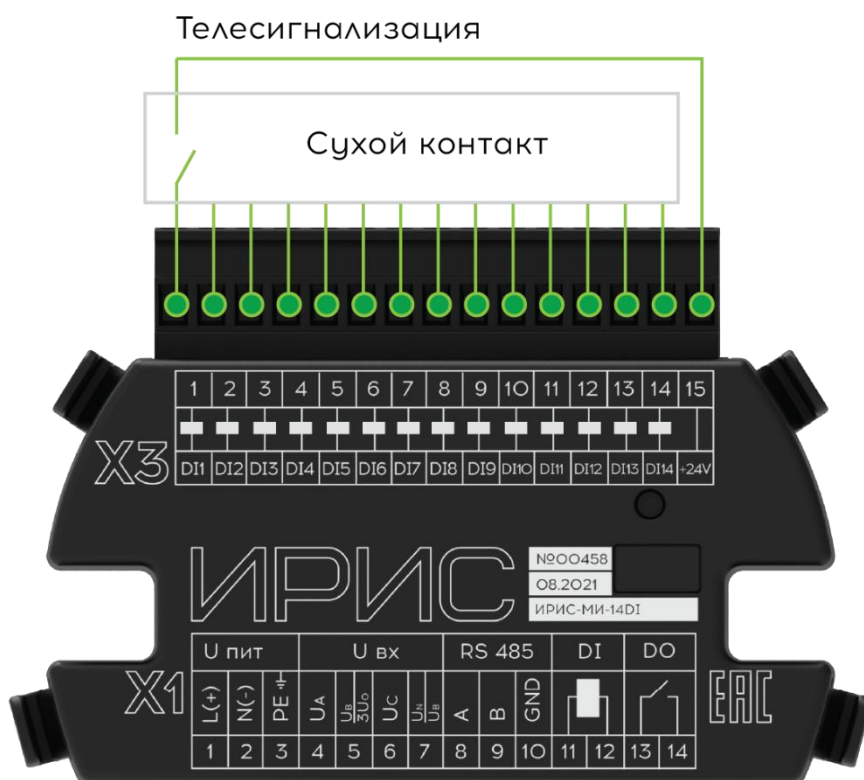
Рисунок 12.6 - Схема подключения рюкзака ИРИС - 14DI
