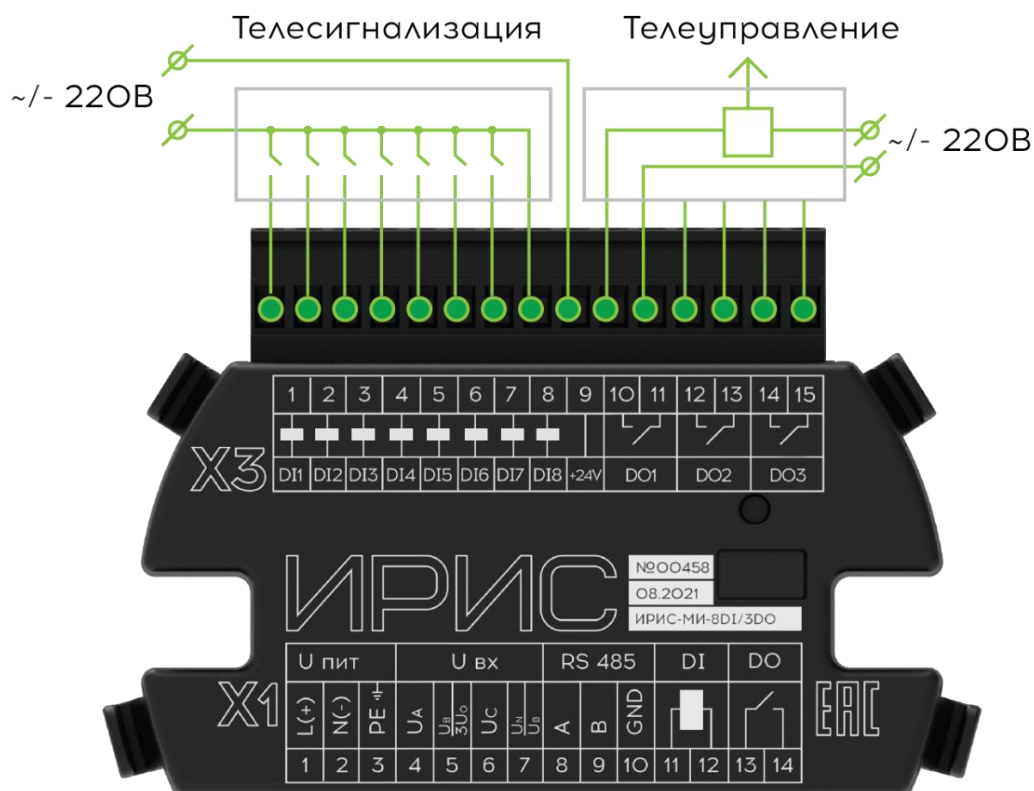
Рисунок 12.8 - Схема подключения рюкзака ИРИС - 8DI/3DO-220V
