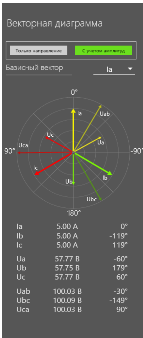
Рисунок 4.6 – Внешний вид векторной диаграммы
