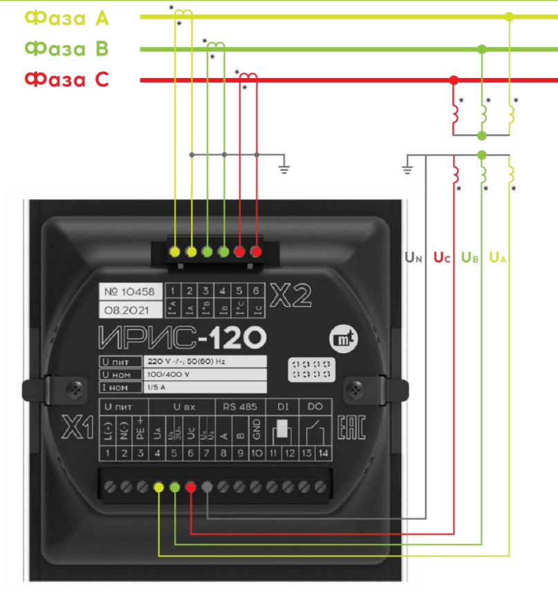
Рисунок 10.2 - Схема подключения устройства с внешними трансформаторами тока и трансформаторами напряжения (ЗТТ, ЗТН)
