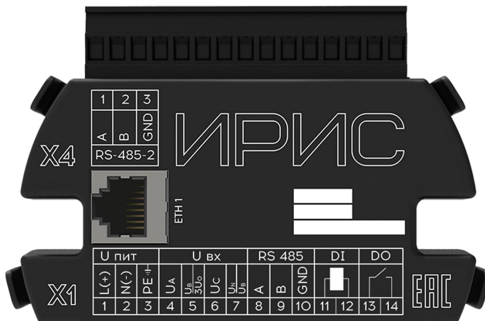
Рисунок 12.10 – Внешний вид рюкзака ИРИС-МИ-ETH
