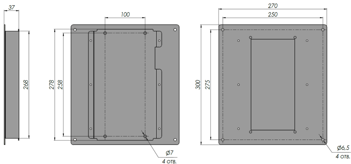
Рисунок П5.6 – Габаритные размеры МТ.АЛТЕЙ.АР.003-01.01
