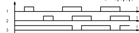
Логическое "И-НЕ"
