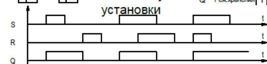
Триггер с приоритетом по сигналу установки
