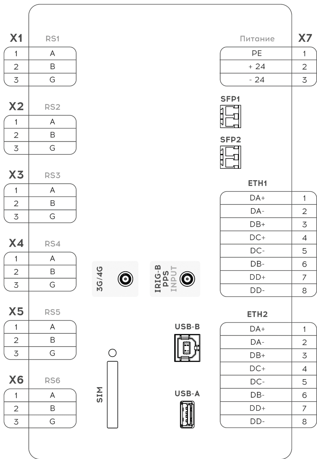
Рисунок Б.11.2 – Схема подключения исполнений GARA-24-B-B-Г
