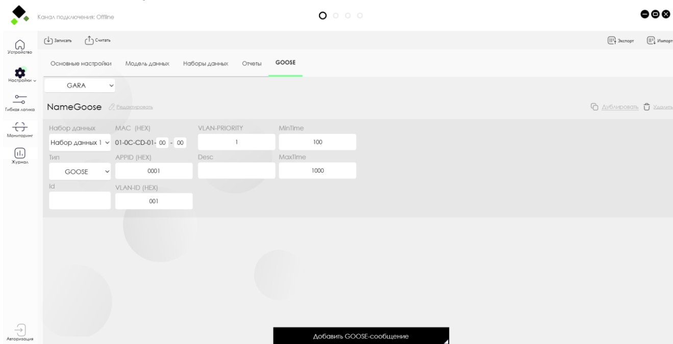
Рисунок 4.17 – GOOSE-сообщения сервера 61850
