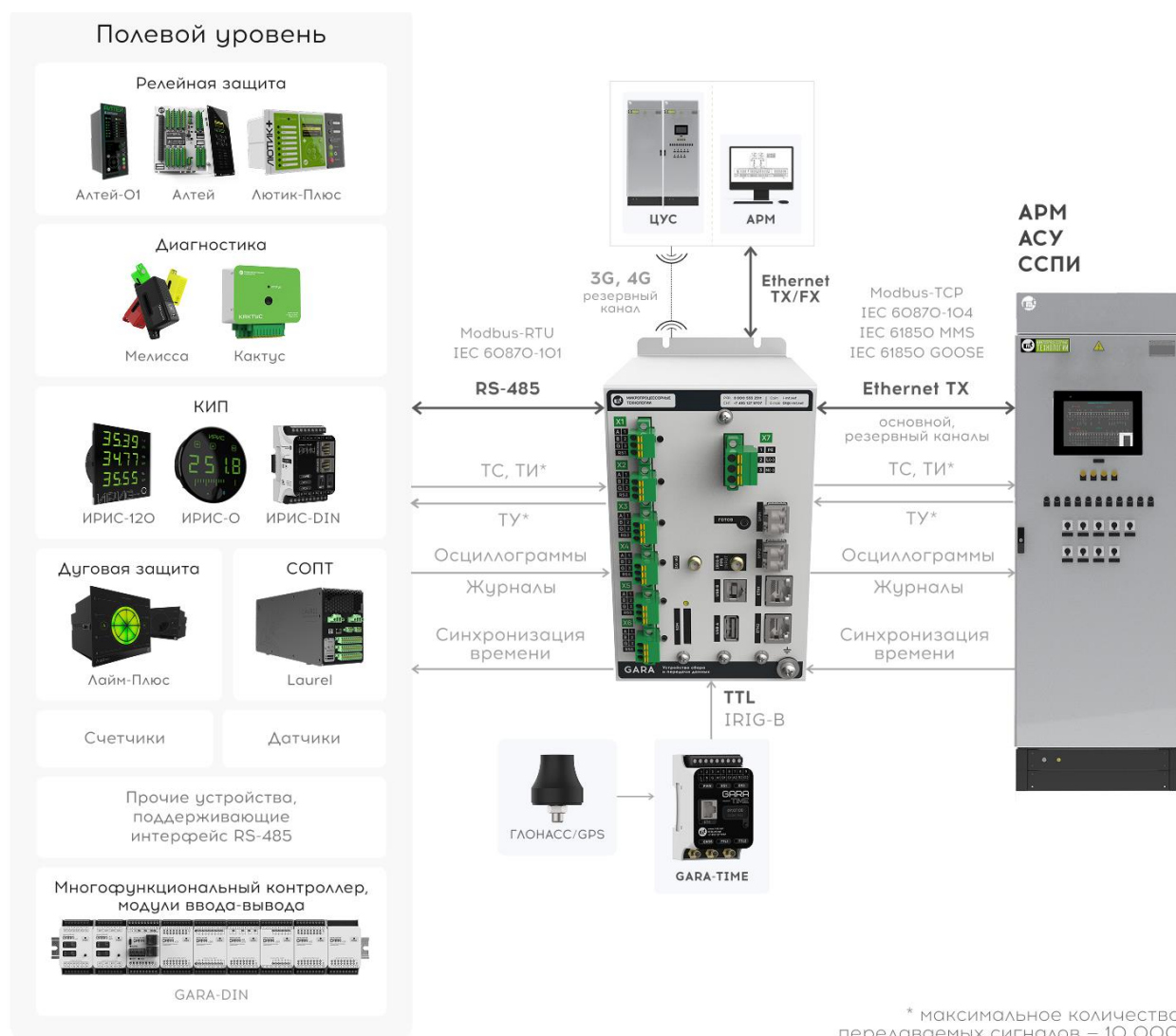
Рисунок 1.1 – Структурная схема системы сбора и передачи данных
