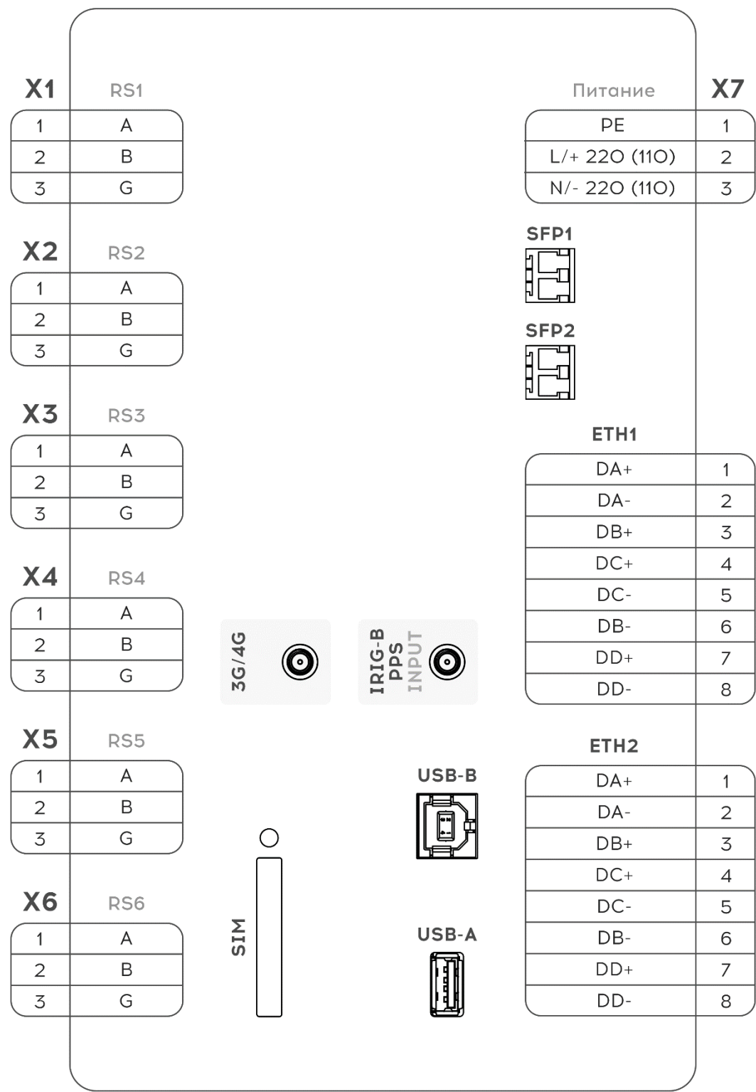
Рисунок Б.11.1 – Схема подключения исполнений GARA-220-B-B-Г
