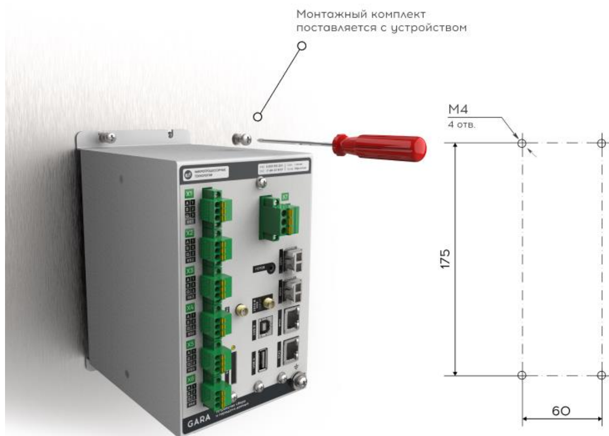
Рисунок А.10.2 – Пример монтажа
