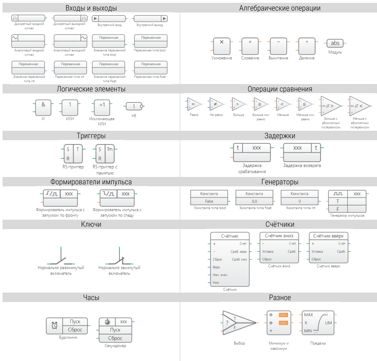
Рисунок 4.26 – Элементы гибкой логики
