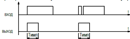
Формирование импульса по положительному фронту
