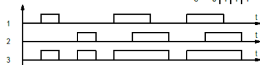
Логическое "ИЛИ"
