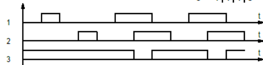
Логическое "И-НЕ"
