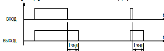
Регулируемая и постоянная задержка на возврат
