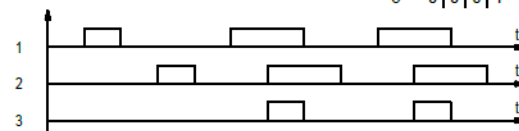
Логическое "И"
