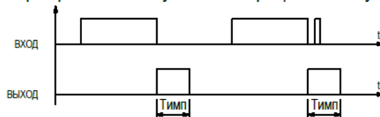
Формирование импульса по отрицательному фронту
